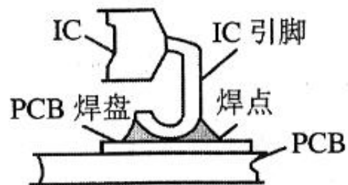
(b) J形引脚
